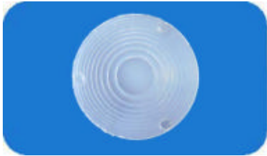
型号：8183 焦距：20 角度：30° 距离比：6:1 尺寸：16.8
