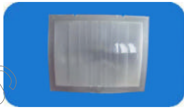
型号：8203-1C 焦距：25 角度：110° 距离：10m 尺寸：44×56.5
